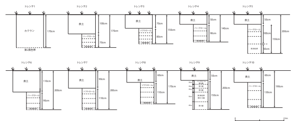
第31図 トレンチ柱状図
