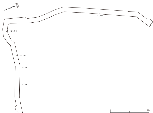
第57図 トレンチ配置図
