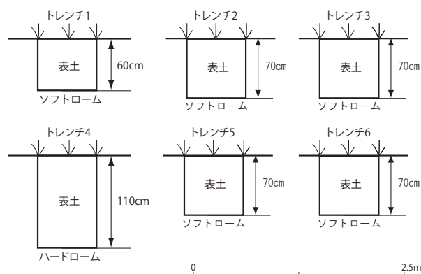
第52図 トレンチ柱状図
