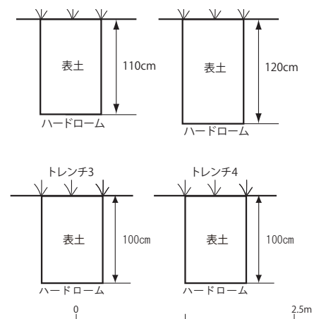
第55図 トレンチ柱状図
