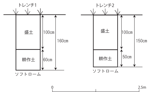
第61図 トレンチ柱状図
