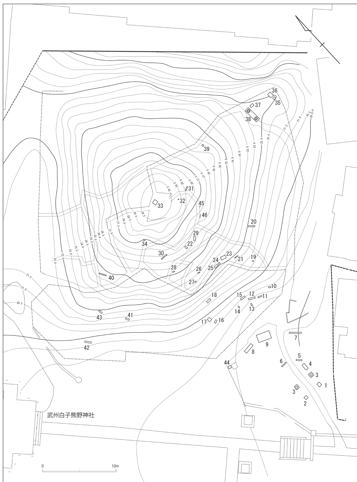
白子富士塚（白子熊野神社）平面図
