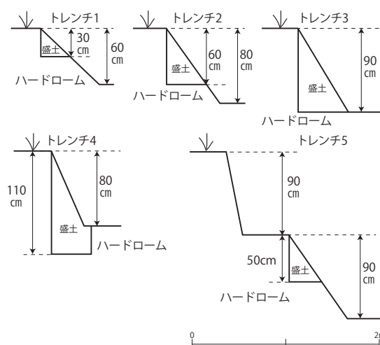
第19図 トレンチ柱状図
