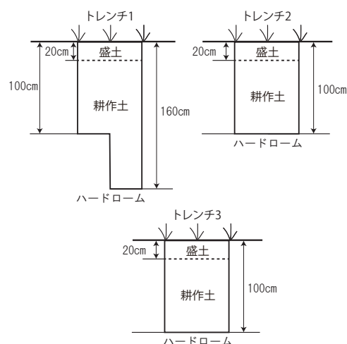
第25図 トレンチ柱状図
