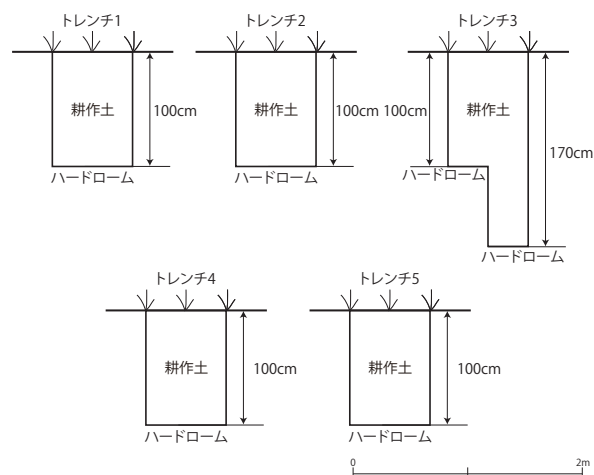
第7図 トレンチ柱状図
