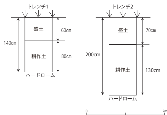
第 51 図 トレンチ柱状図
