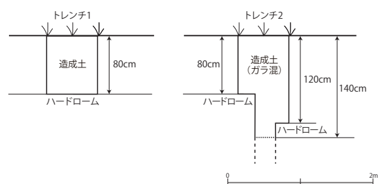
第40図 トレンチ柱状図
