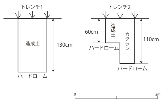
第54図 トレンチ柱状図
