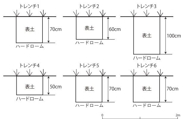
第10図 トレンチ柱状図
