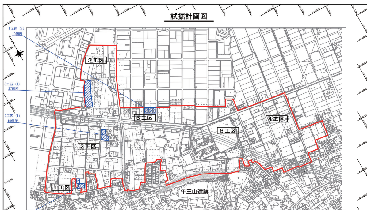
第 44 図 調査地点位置図
