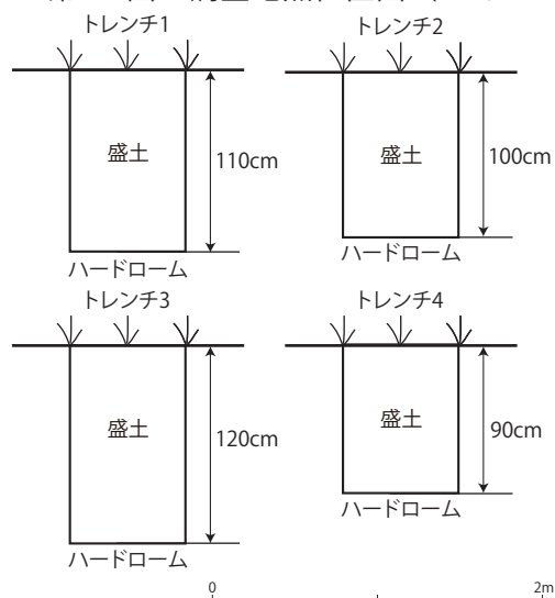
第13図 トレンチ柱状図
